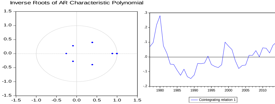
Şekil 1: AR Karakteristik Polinomunun Ters Köklerinin Birim Çember İçindeki Konumu ve Eşbütünleşme Grafiği
