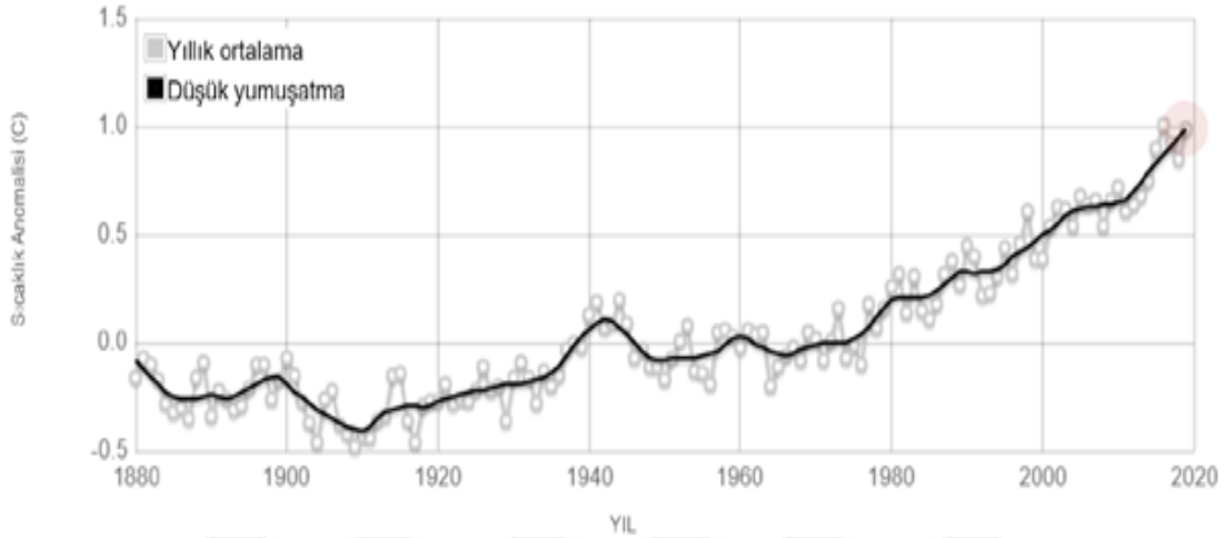
Grafik 1.1. Küresel kara-okyanus sıcaklık endeksi (NASA / GISS, 2020).
