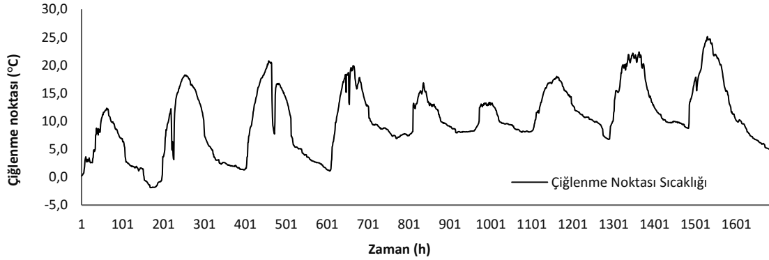
Şekil 10 Sera bilgisayarı ile hesaplanan çiğlenme noktası sıcaklığı değerleri
