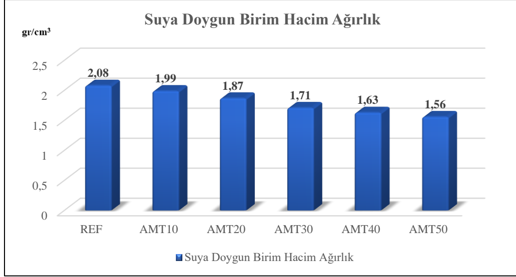
Şekil 4.1. Numunelerin suya doymun birim hacim ağırlık değerleri
