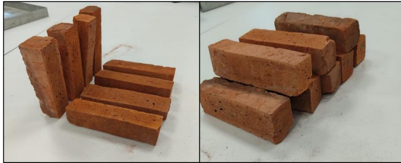
Şekil 3.3. Atık mermer tozu katkılı tuğla numunesi
