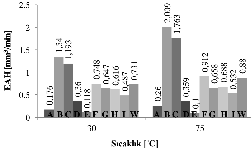
Şekil 11. Farklı karışımlar içinde dönmeyen elektrotla işlemede EAH-sıcaklık değişimleri (The EWR-temperature variations at machining with non-rotating electrode in different mixtures)
