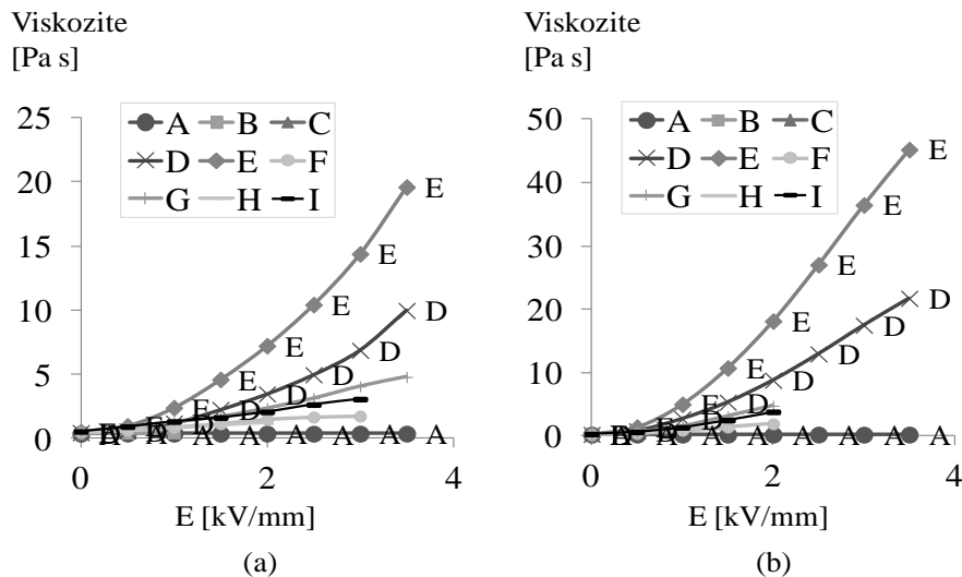
Şekil 7. Dielektrik karışımların viskozite-elektrik alan değişimleri: a) 30°C ve b) 75°C (The viscosity-electric field variations of dielectric mixtures: a) 30°C and b) 75°C)
