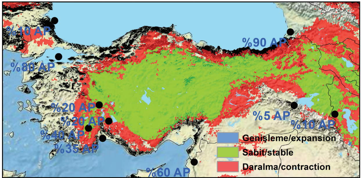
Şekil 11. Son Buzul Maksimum'dan günümüze Anadolu yer sincabının ( Spermophilus xanthoprimum ) coğrafi dağılımındaki değişiklikler. Siyah noktalar Son Buzul Maksimum'daki ağaç poleni (AP) yüzdeleri (Şenkul and Doğan 2013'den), siyah alanlar ise günümüzde orman örtüsünün %50'nin üzerinde olduğu yerleri gösterir (Forest Europe 2011'e dayanarak çizilmiştir).
