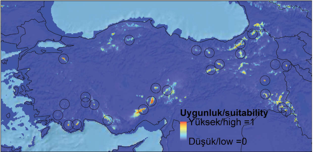
Şekil 6. Son Buzul Maksimum iklimsel koşulları altında Anadolu’da buzul gelişimi için iklimsel olarak uygun alanlar. Sonuçlar, ekolojik niş modellemesi yaklaşımı kullanılarak, MAXENT yazılımındaki (versiyon 3.3.3k) maksimum entropi makine öğrenme algoritması ile elde edilmiştir (bkz. ana metin). Buzulların coğrafi dağılımı (çemberler, n = 27), Sarıkaya vd. (2011)’den alınmıştır. İklimsel veri, yaz ve kış ortalama sıcaklıklarını ve yağışlarını içerir ve WorldClim veri tabanından (versiyon 1.4, www.worldclim.org ) elde edilmiştir. Bu veri, üç farklı küresel iklim modeline dayanır: CCSM4, MIROC-ESM ve MPI-ESM-P. Karasal alanlar, Son Buzul Maksimum ile günümüz arasında farklıdır.
